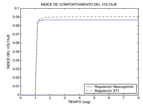
Figura 4.11. Índice de comportamiento del voltaje en terminales.
