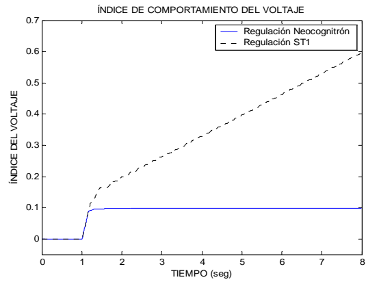
Figura 4.17. Índice de comportamiento del voltaje en terminales.
