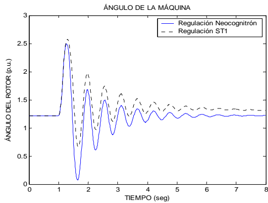
Figura 4.30. Comportamiento del ángulo de la máquina ante una falla de 9 ciclos de duración.
