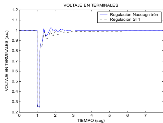
Figura 4.10. Comportamiento del voltaje en terminales ante una falla de 9 ciclos de duración.
