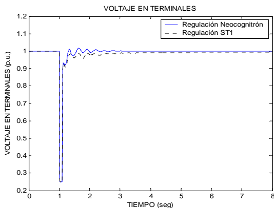
Figura 4.76. Comportamiento del voltaje en terminales ante una falla de 6 ciclos de duración.
