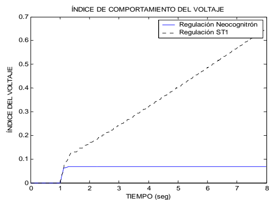
Figura 4.65. Índice de comportamiento del voltaje en terminales.
