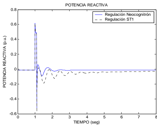
Figura 4.44. Comportamiento de la potencia reactiva ante una falla de 6 ciclos de duración.
